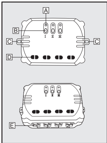
A: LED-indicator B: Verbindingsknop C: Bevestigingspunten D: Klemmschroeven E: Stroomaansluiting
